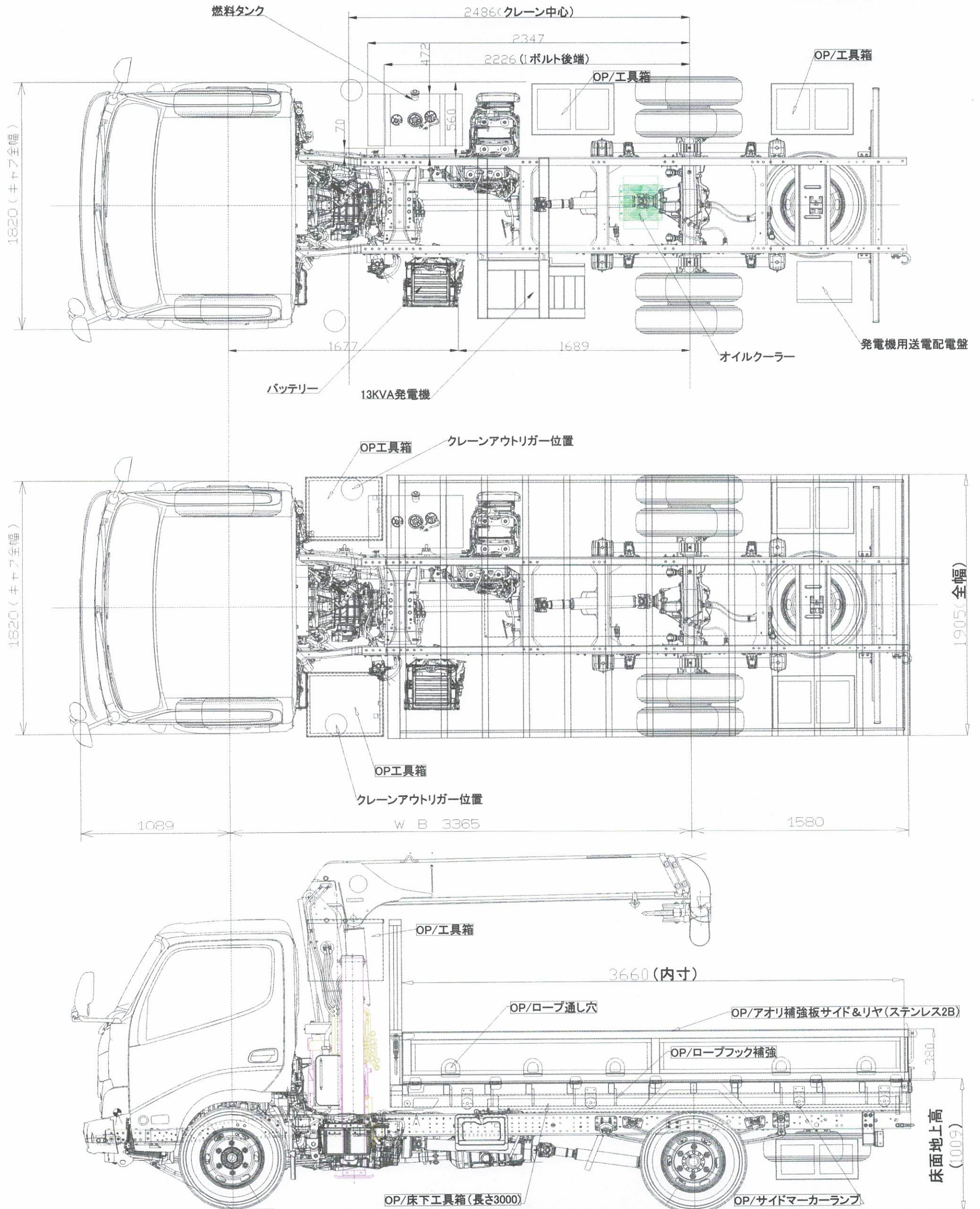
(床下レイアウト図)
